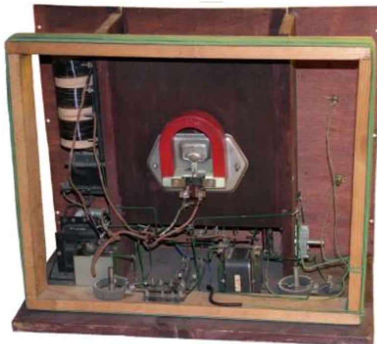
Innenansicht bei abgenommener Lautsprechermembran
